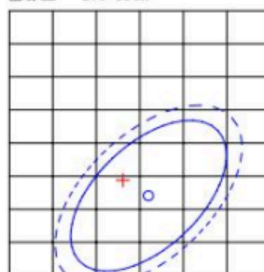
CIE1931色品图
