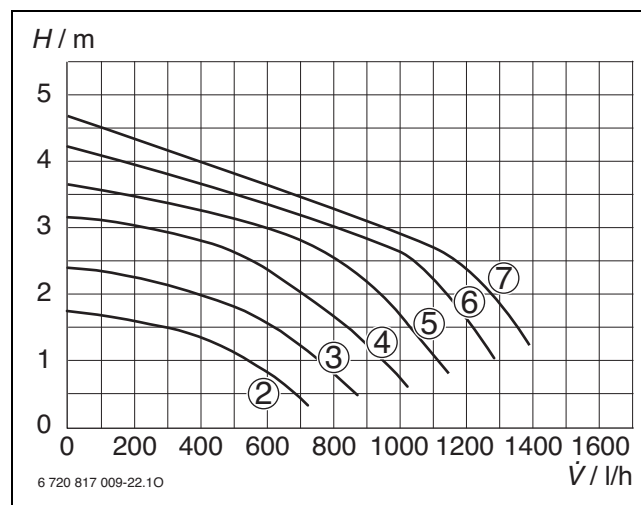
Fig. 31 Curvas características de las bombas
