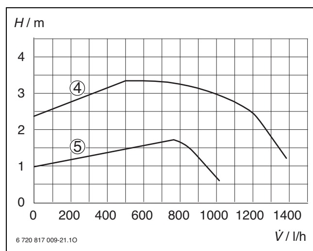
Fig. 30 Presión proporcional
