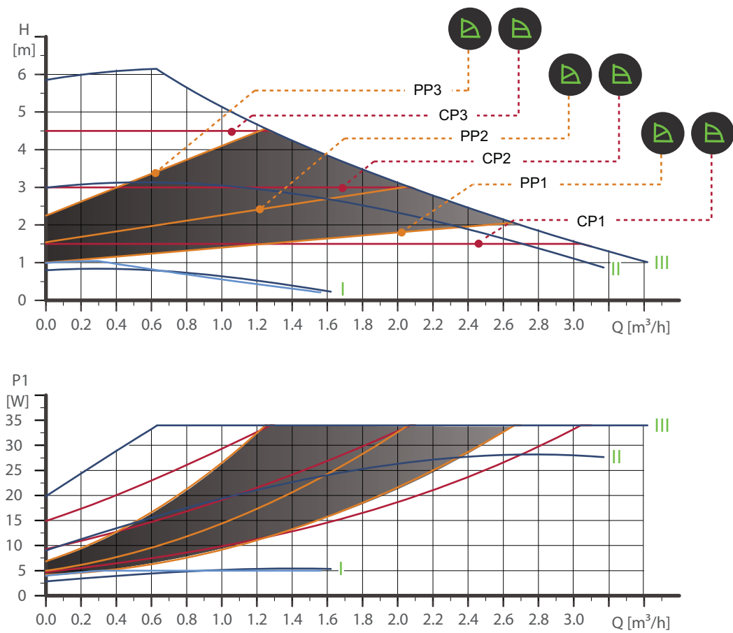
Abb. 32 ALPHA2 XX-60
