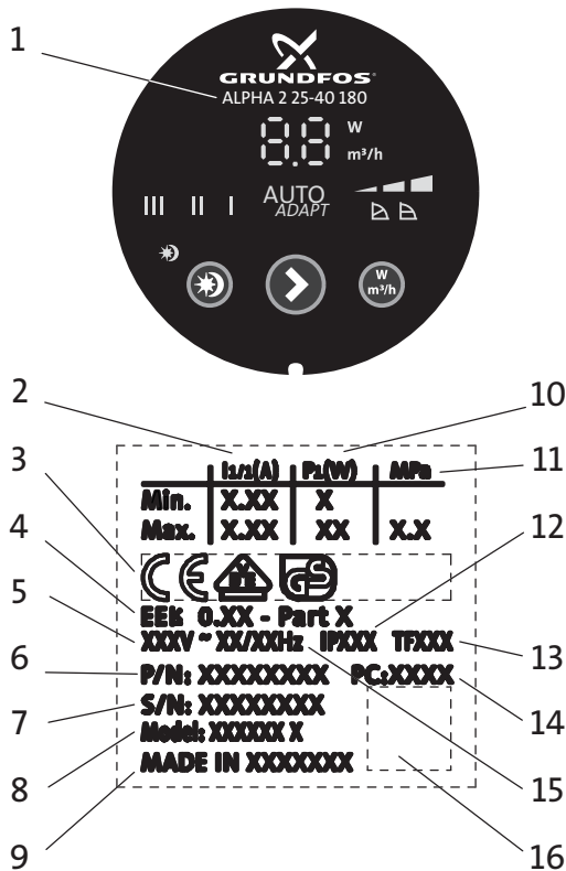
Abb. 2 Typenschild
