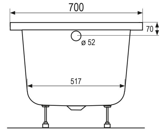
CAMARGUE ORLANDO 26062149, 150x70 cm Einbauhöhe: ab 58,5 cm
