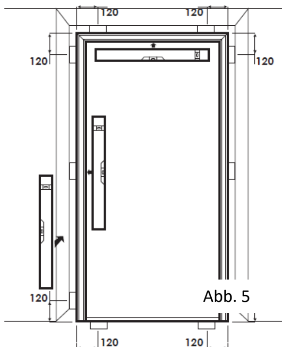
Montage mit den Schrauben
