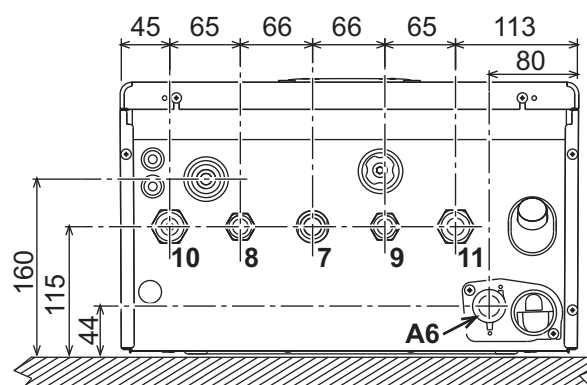
fig. 56- Vista inferior
