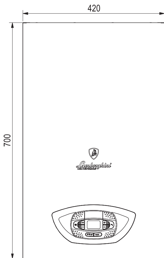
fig. 53- Vista frontal
