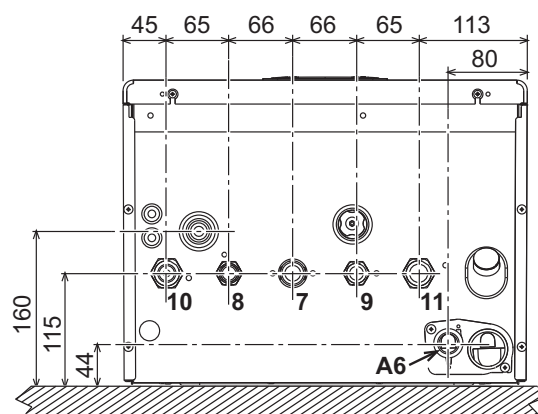
fig. 55- Vista inferior
