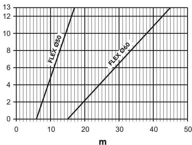
fig. 26- Gráfica para determinar el valor de SC04
