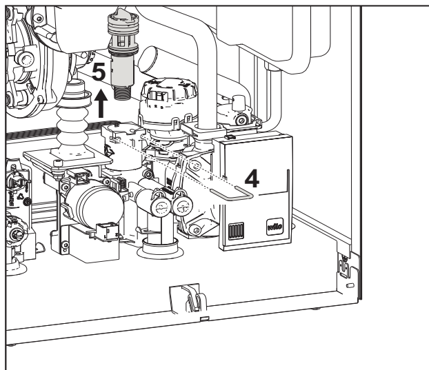
fig. 48- Caudalímetro
