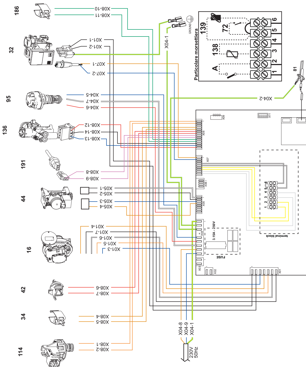
fig. 61- Esquema eléctrico
