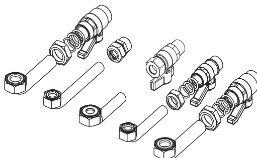
fig. 18- Kit hidráulico
