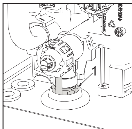
fig. 17- Válvula de seguridad con grifo de descarga
