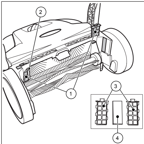
Rys. 12: Wymowanie filtra pyłowego
