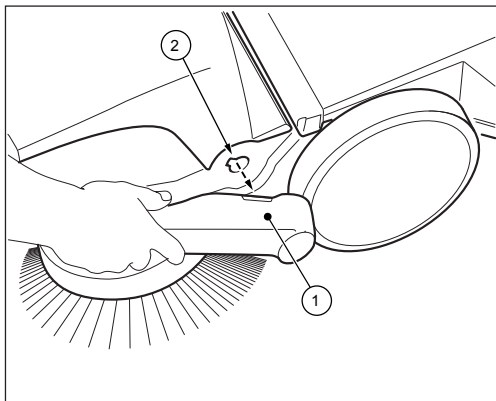
Kuva 14: Työntöaisan irrottaminen (SWP 577)
