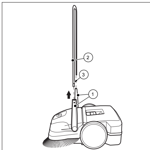
Abb. 13: Schiebebügeldemontage (SWP 475)
