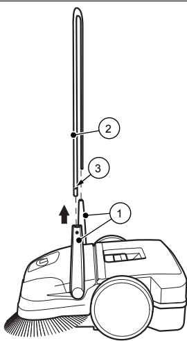
Illustration 13 : Démontage de l'arceau rétractable (SWP 475)
