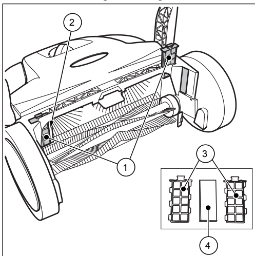
Fig. 12: Støvfilter fjernelse
