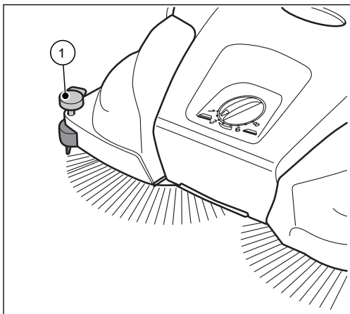
Рис. 10: Установка прижима
