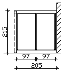
Bemassung
