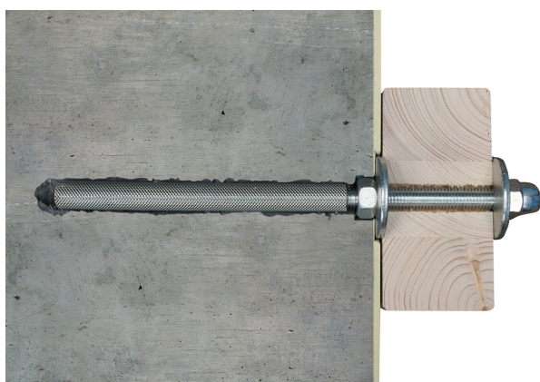
Querschnitt Wandbefestigung
