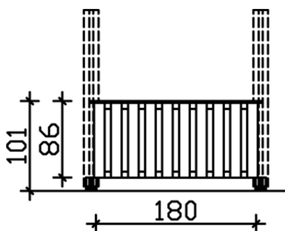
Bemassung
