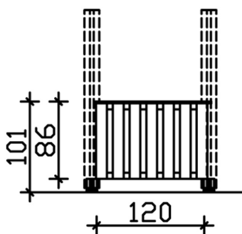
Bemassung
