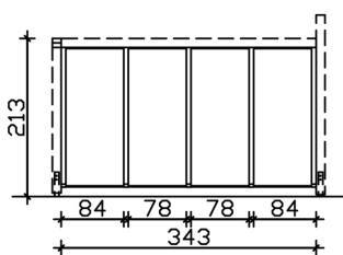
Bemassung
