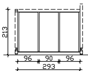
Bemassung
