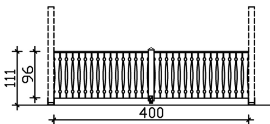
Bemassung
