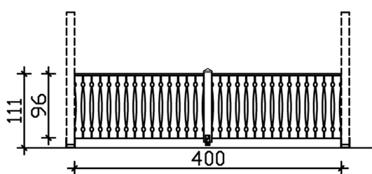
Bemassung
