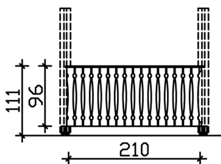
Bemassung
