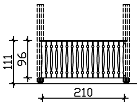
Bemassung
