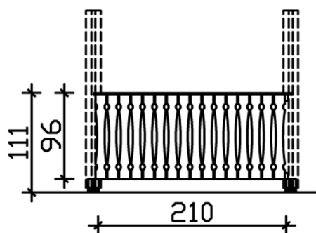
Bemassung
