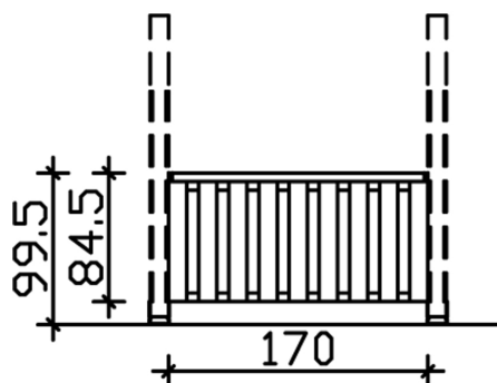
Bemassung
