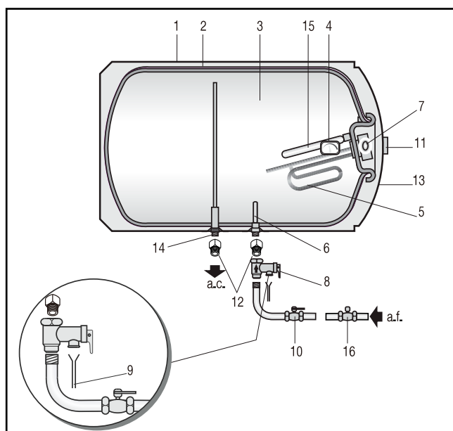
Figura 6 (Instalación horizontal)
