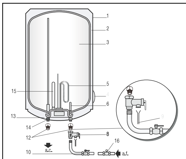
Figura 5 (Instalación vertical)
