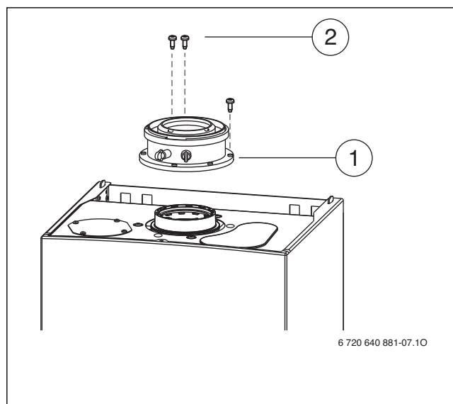
Fig. 31 Colocar el accesorio de gases quemados
