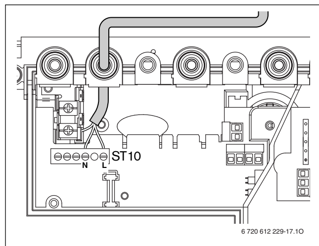
Fig. 39 Regleta de conexión de tensión de alimentación ST10
