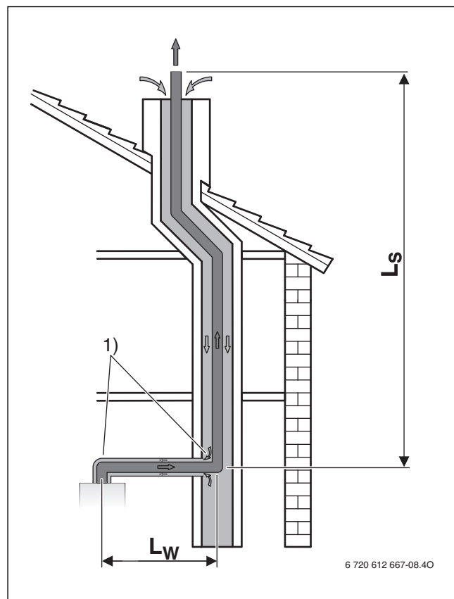
Fig. 16 Conducción de gases en chimenea según C 93
