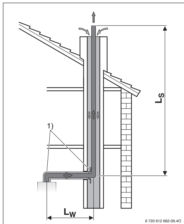
Fig. 15 Conducción de gases en chimenea según C 93
