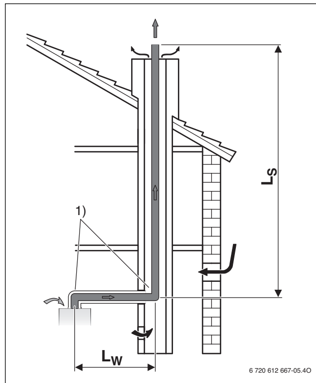
Fig. 11 Conducción de gases en chimenea según B 33
