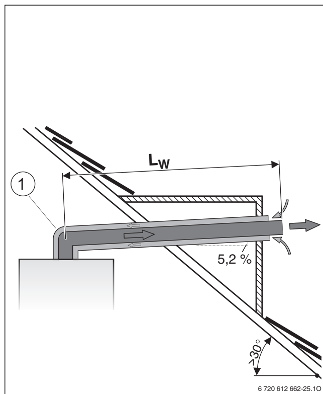
Fig. 19 Conducción de gases horizontal según C 33 (Ø 80/125 mm)
