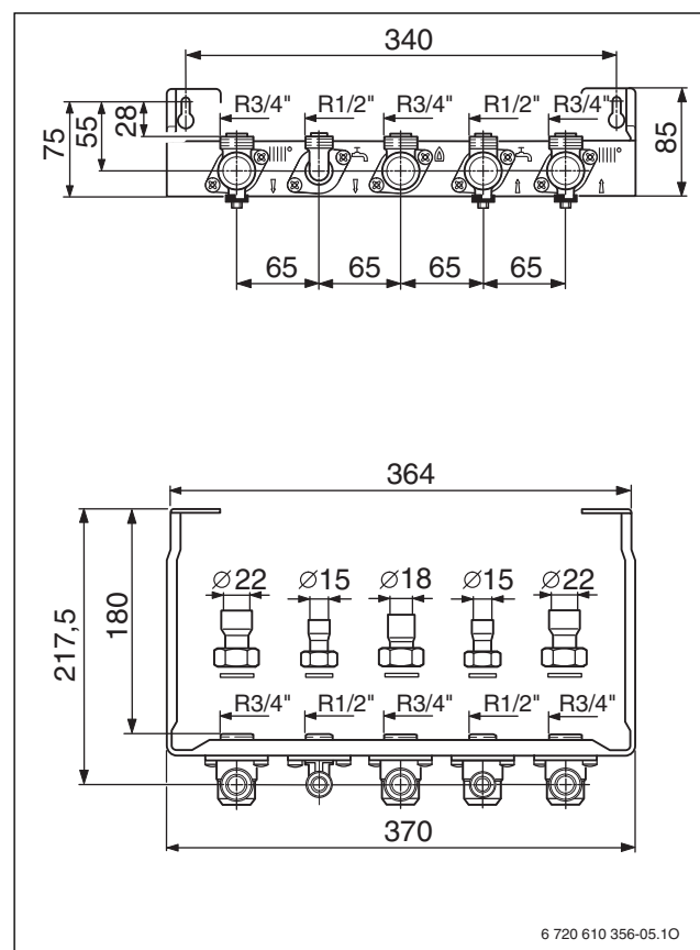
Fig. 24 Placa de conexión para montaje
