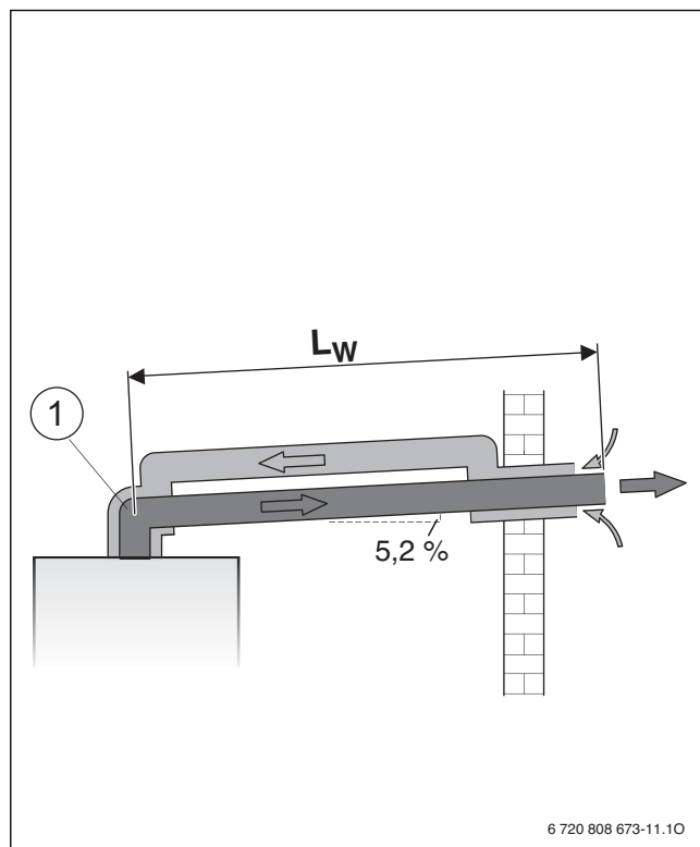
Fig. 20 Conducción de gases horizontal según C 13
