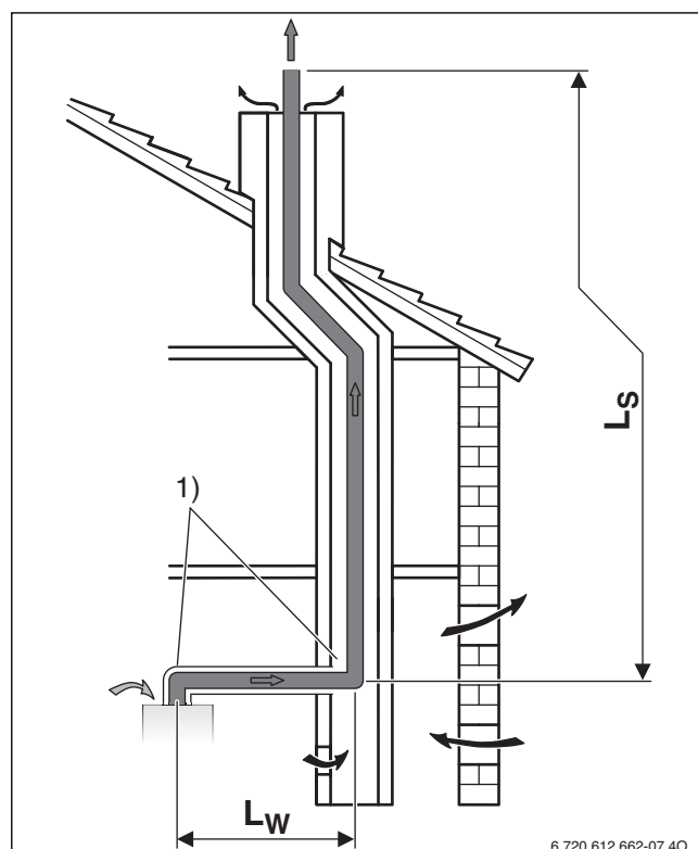
Fig. 12 Conducción de gases en chimenea según B 33
