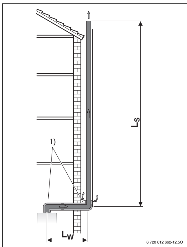
Fig. 21 Conducción de gases en la fachada según C 53
