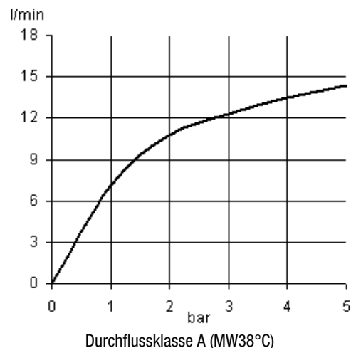
Durchflussdiagramm
