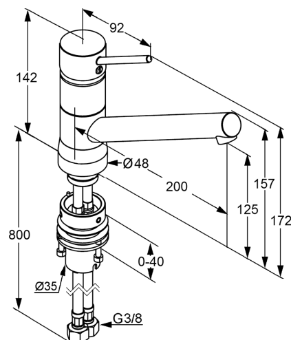
Maßzeichnung
