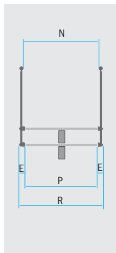
Vorderansicht mit Geländer auf 2 Seiten
