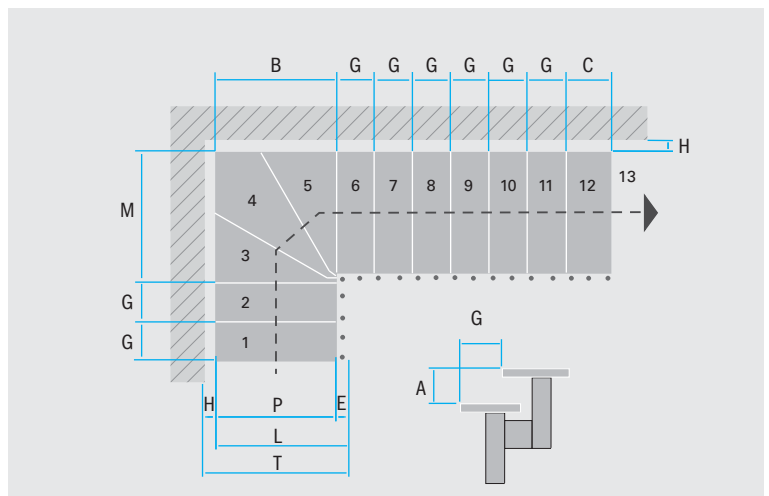
Grundriss mit Abmessungen
