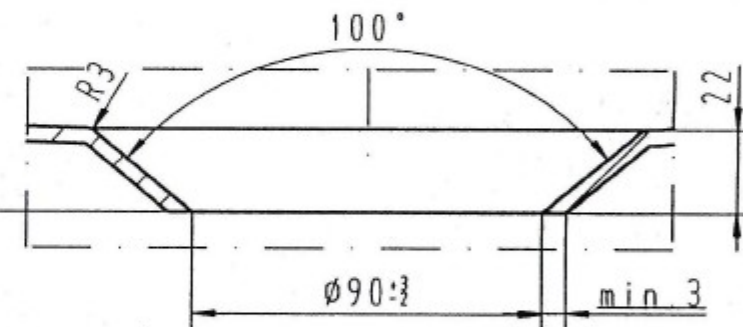
Einzelheit "Y" (M1:2)
