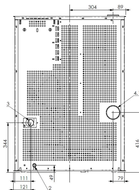
Abmessungen Pelletofen AITANA
