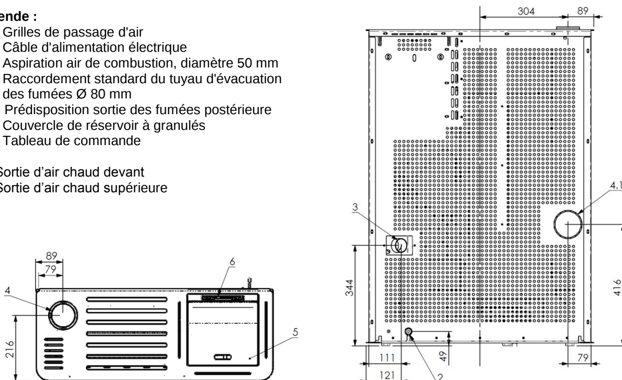
Dimensions du poêle à granulés AITANA
