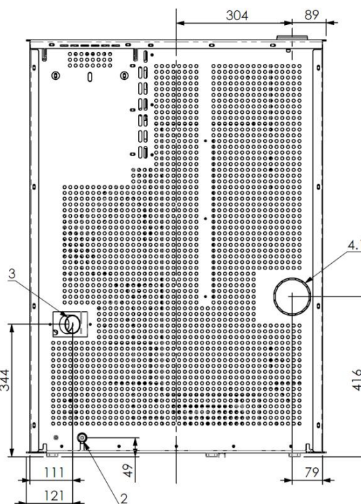
Medidas de la estufa de pellets AITANA
