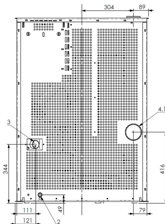
Ingombri stufa pellet AITANA
