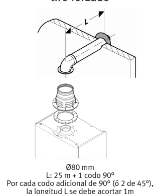
Configuración tipo B22 tiro forzado
