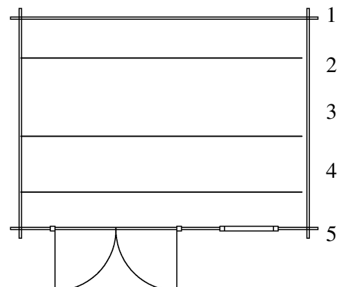
Grundriss und Fundamentplan (5 Fundamenthölzer)
