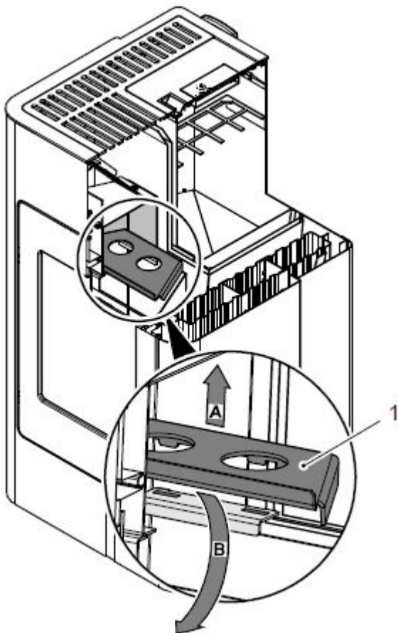
Abbildung 8a: Demontage der Zugumlenkung
