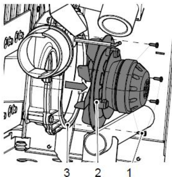
Abbildung 9: Saugzuggebläse
