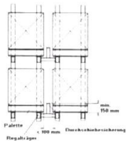
Abb. 8a: Durchschiebesicherung
