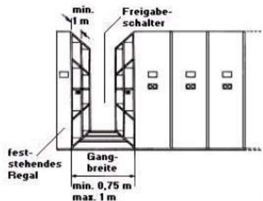
Abb. 16: Sicherung durch Freigabeschalter.
