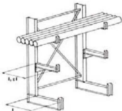
Abb. 10: Beispiel für die Ausführung von Kragarmregalen
