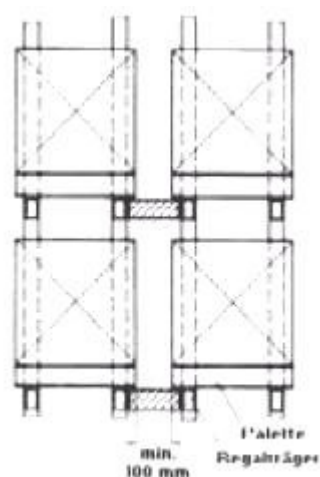
Abb. 8b: Sicherheitsabstand
