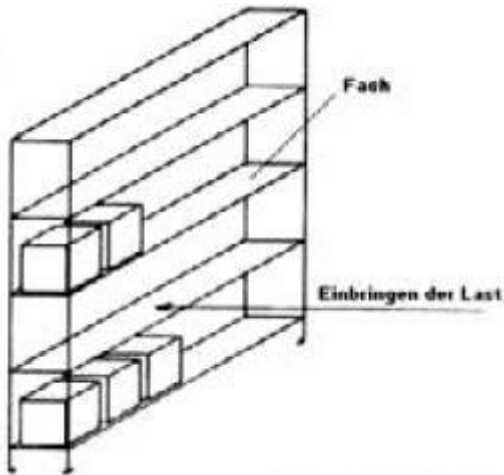
Abb. 9a: 4 Fächer = Feld eines Einfachregals
