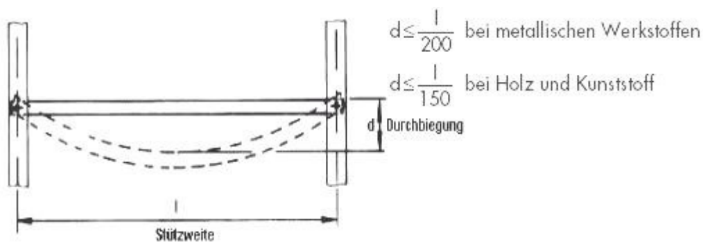
Abb. 1: Höchstzulässige Durchbiegung der tragenden Elementen von Lagereinrichtungen.
