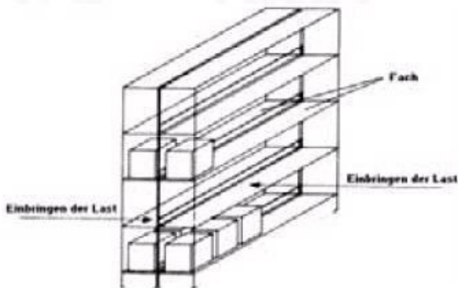
Abb. 9b: 8 Fächer = Feld eines Doppelregals
