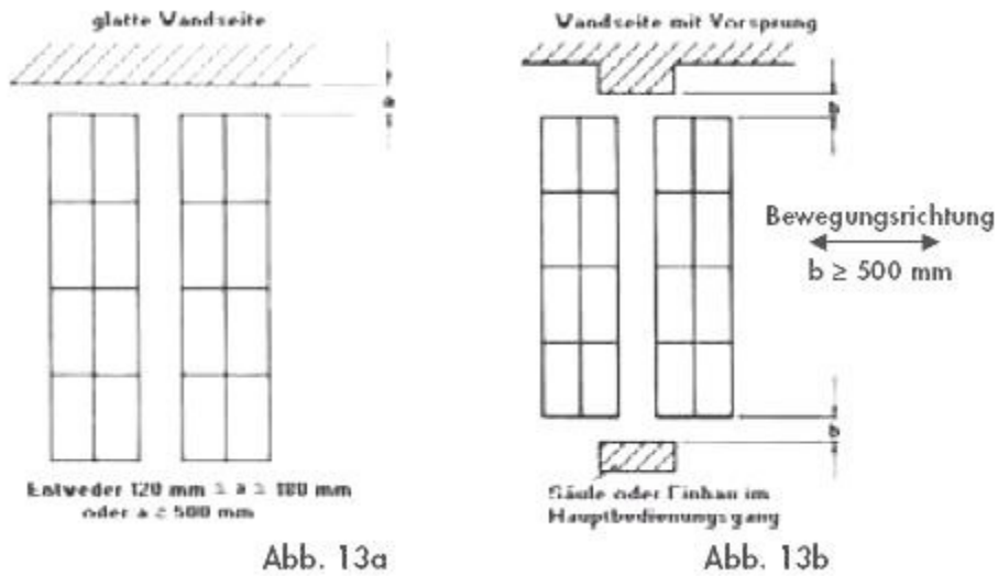
Abb. 13: Wandabstände verfahrbarer Regale und Schränke.
