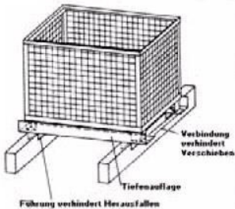
Abb. 6: Beispiel für einsatz und Gestaltung von Tiefenauflagen.
