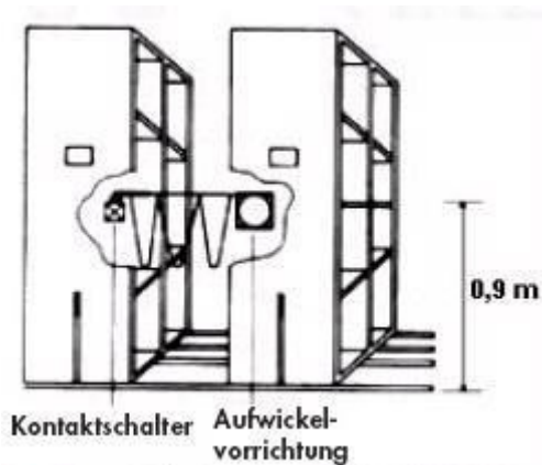
Abb. 15: Beispiel einer Seilzugsicherung bei geschlossenem Steuerstromkreis.
