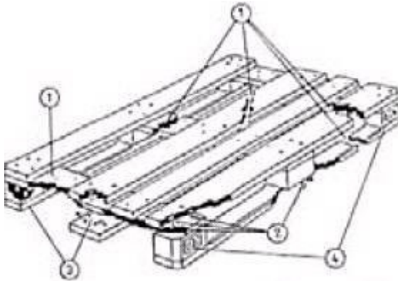
Abb. 18: Schäden oder Mängel an Flachplatten nach UIC 435-4 VE
