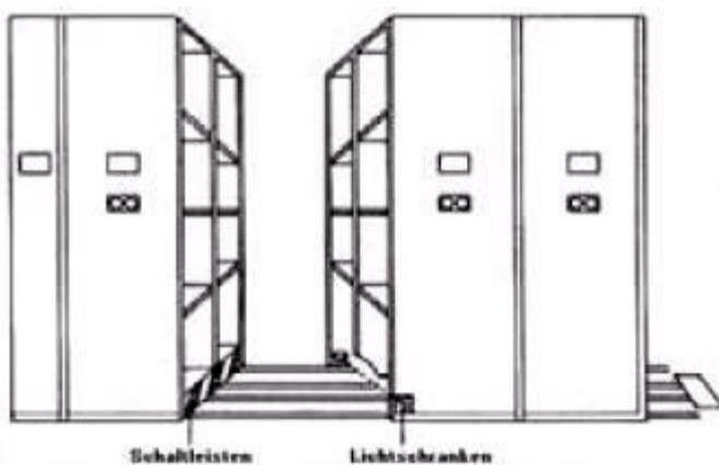
Abb. 14: Sicherung durch Schaltleisten oder Lichtschranken.
