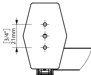
FIJACIÓN PARED WALL FIXATION
