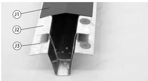
Firststabdeckung (J1) roof ridge cover (J1) Firstträger oben (J2) upper roof ridge beam (J2) Firstträger unten (J3) lower roof ridge beam (J3) couverture de faîtière (J1) copertura colmo (J1) poutre de faîtage sup. (J2) supporto colmo superiore (J2) poutre de faîtage inf. (J3) supporto colmo inferiore (J3)
