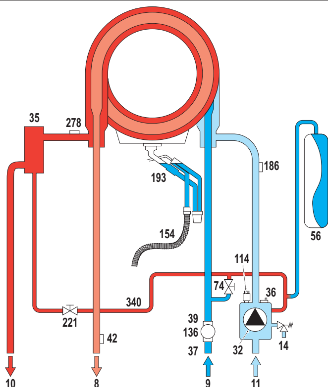
fig. 27 - Circuito hidráulico
