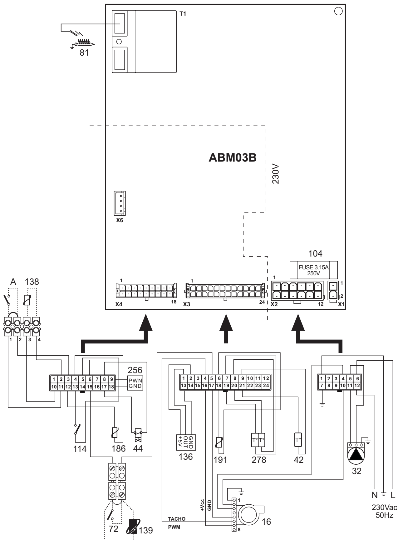
fig. 30 - Esquema eléctrico
