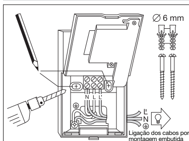
Ligação dos cabos por montagem embutida
