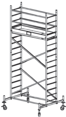
Baugruppennr. Arbeitshöhe: 5,30 m 2203 Gerüsthöhe: 4,30 m Artikel Nr. Standhöhe: 3,30 m 910134 xxxxxx
