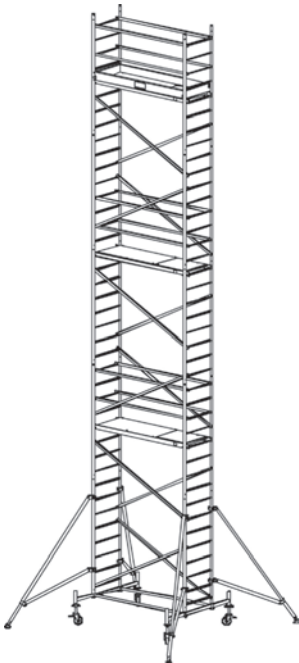
Baugruppennr. Arbeitshöhe: 11,30 m 2209 Gerüsthöhe: 10,30 m Artikel Nr. Standhöhe: 9,30 m 910196 xxxxxx
