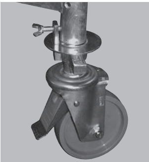
Fahrrolle gebremst
