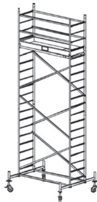
Baugruppennr. Arbeitshöhe: 6,30 m 2204 Gerüsthöhe: 5,30 m Artikel Nr. Standhöhe: 4,30 m 910141 xxxxxx
