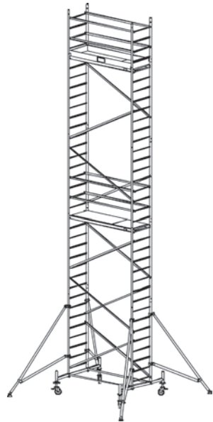
Baugruppennr. Arbeitshöhe: 10,30 m 2208 Gerüsthöhe: 9,30 m Artikel Nr. Standhöhe: 8,30 m 910189 xxxxxx
