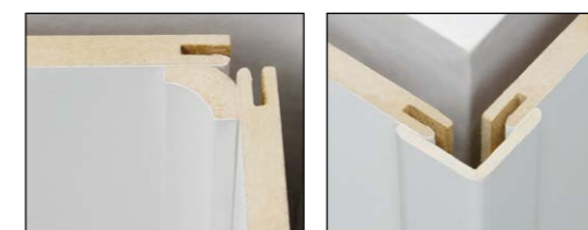
Hohlkehlleiste 16 x 16 x 2600 mm 22 x 22 x 2600 mm
