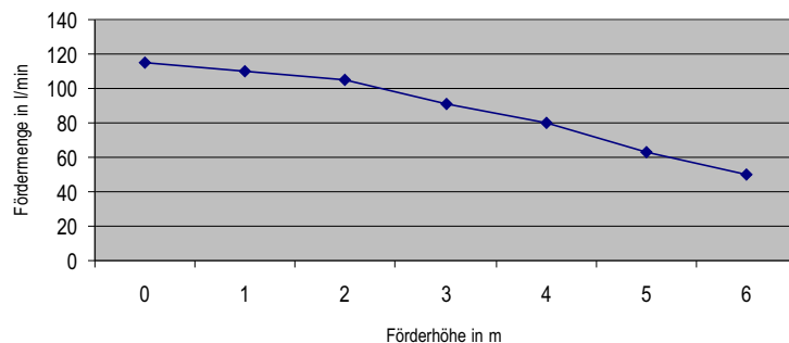
Förderkurve WATERSAN 6
