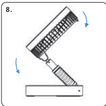
Plegado 2: con el dispositivo de bloqueo liberado, baje el tubo hasta su posición original y pliegue el ventilador.
