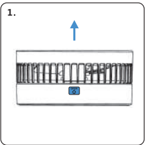
Con el ventilador plegado, tire hacia arriba desde la posición «OPEN», luego ábralo.
