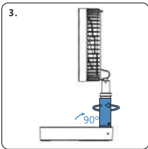
Levante el ventilador 90° hasta la vertical y luego gire el dispositivo de bloqueo en sentido horario para bloquearlo una vez abierto.
