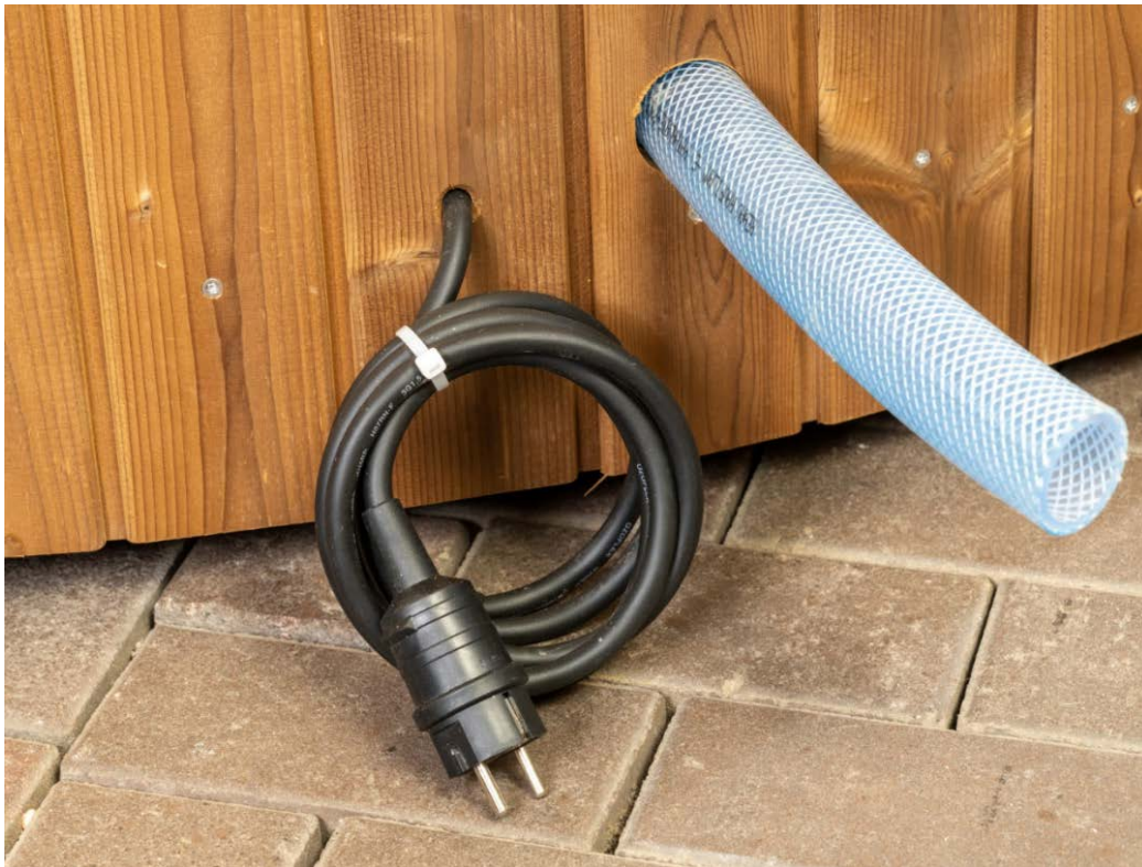
Abbildung 27: Darstellung des 230 V-Schuko-Steckers des Hot Tubs (rechts daneben: Vorbereitung für die Sandfilteranlage (Wasser-Rücklauf zur Sandfilteranlage))
