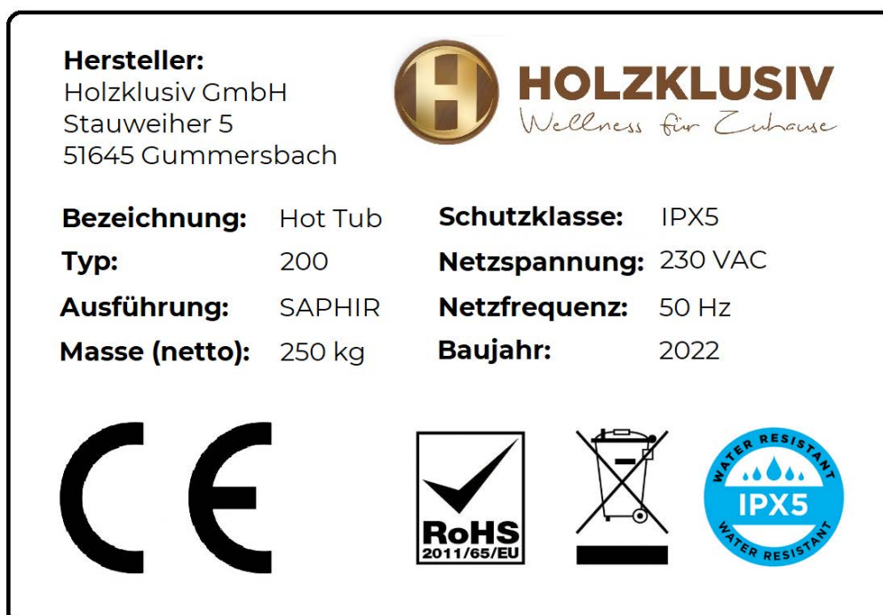
Abbildung 7: Typenschild, dargestellt für die Ausführungsvarianten SAPHIR und dem Typen 200
