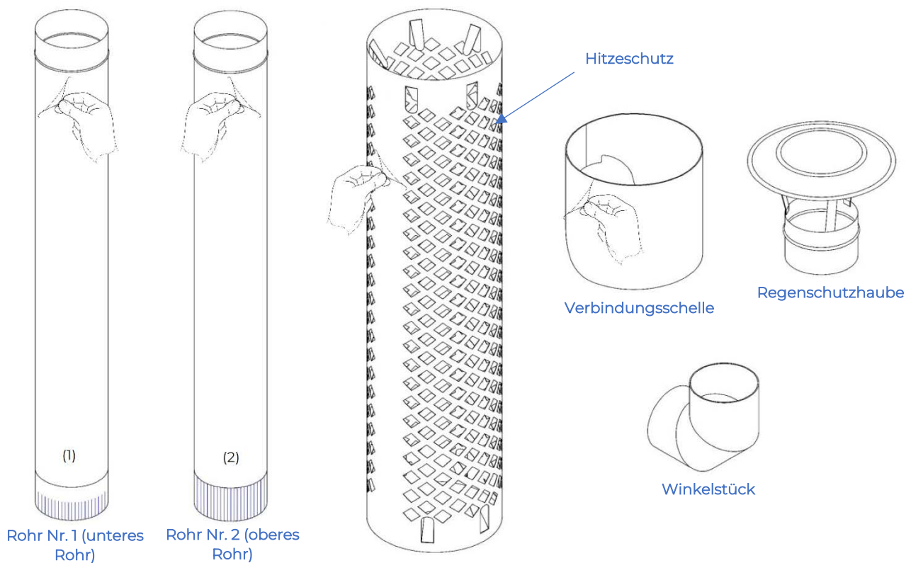
Abbildung 14: Lieferumfang des Abzugsrohres
