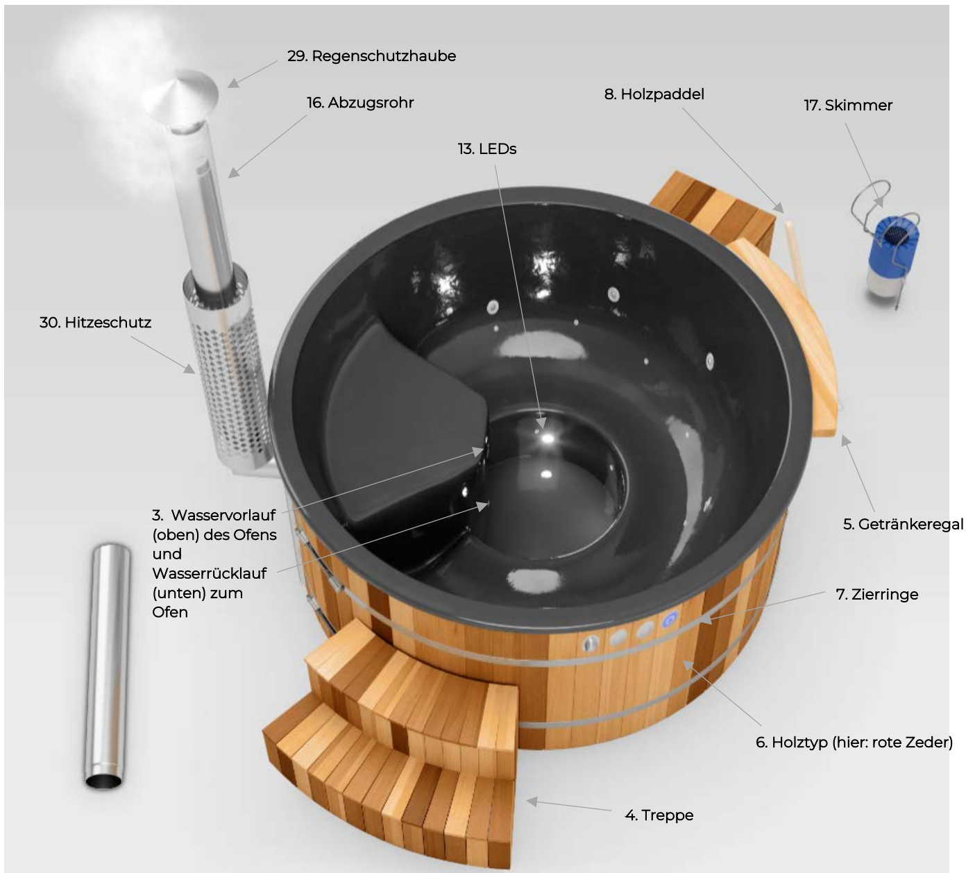
Abbildung 6: Isometrische Ansicht des Hot Tubs, Ausführungsvariante „SAPHIR“
