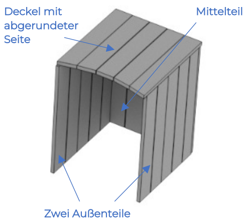
Abbildung 20: Lieferumfang, Verschrauben der Wände, Deckel auflegen
