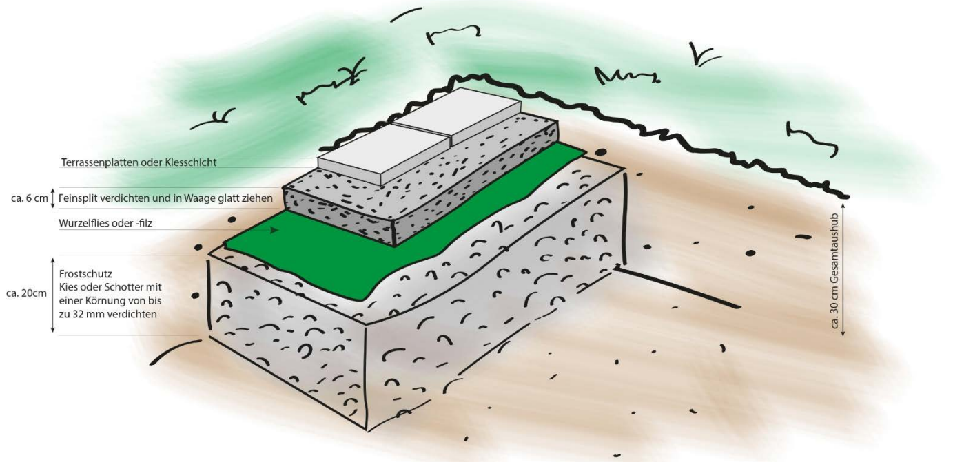
Abbildung 13: Beispielhafte Vorbereitung des Aufstellortes
