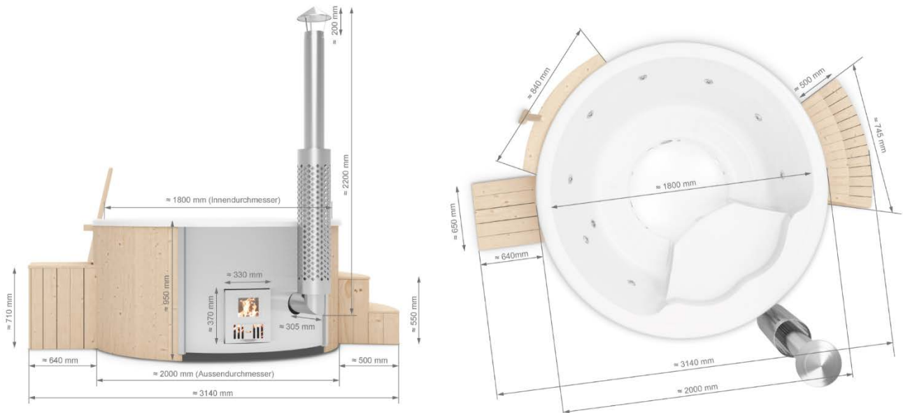
Abbildung 8: Maße des Hot Tubs 180, Ausführungsvariante „SAPHIR“
