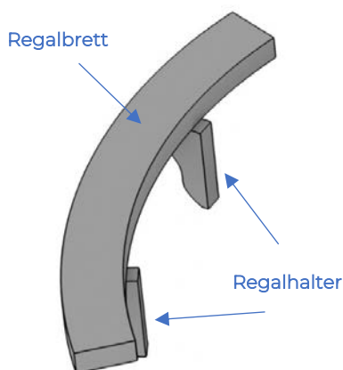
Abbildung 18: Lieferumfang, Markierung der Montageposition der Oberkante der Regalhalter, Positionierung des Regalbretts
