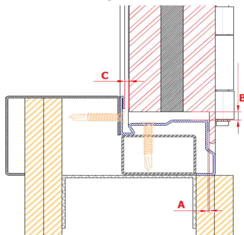
DETALLE 5
