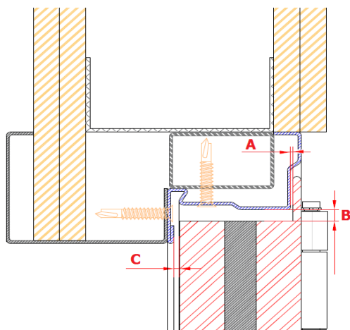
DETALLE 4
