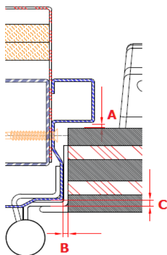
DETALLE 2
