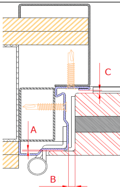
DETALLE 6
