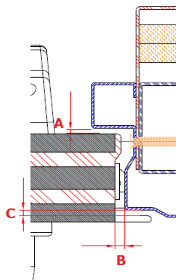
DETALLE 3
