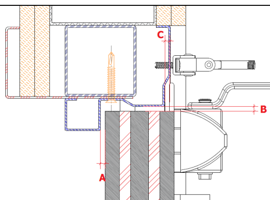
DETALLE 1
