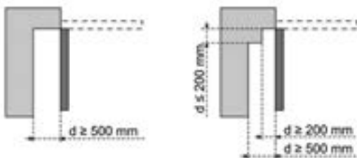
Figuur 4 - Veiligheidsafstand
