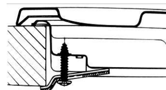
Posición del gancho H=40mm tope
